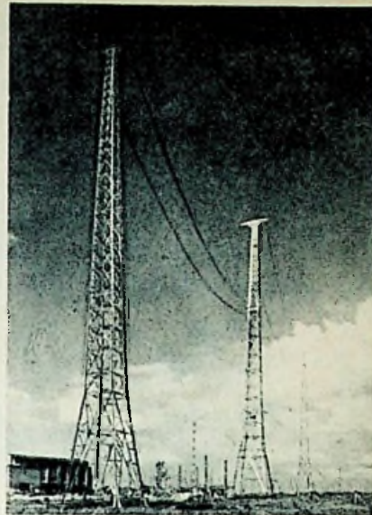
Het antennepark van het nieuwe zendcentrum.
