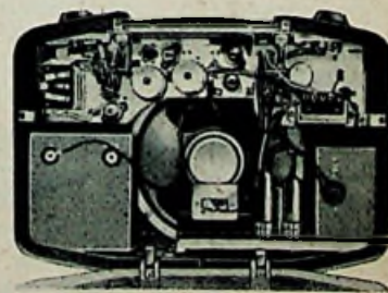
Pye P 65 MBQ met geopende achterwand.
